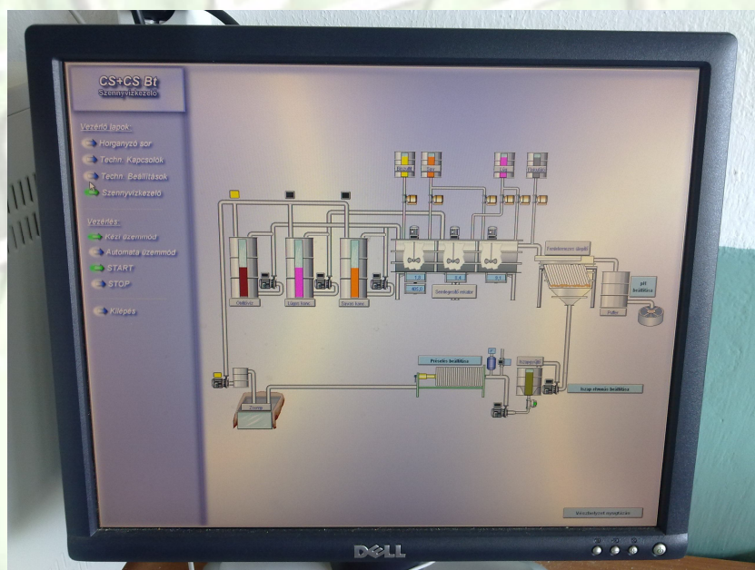
Szennyvízkezelő berendezés folyamatmegjelenítője
